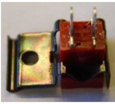
Датчик температуры LEJ (36200690) Lamborghini, Италия (F398D1350)
